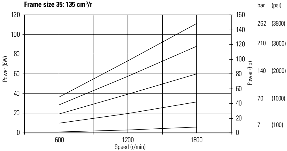
Frame size 35: 135 cm 3 /r
