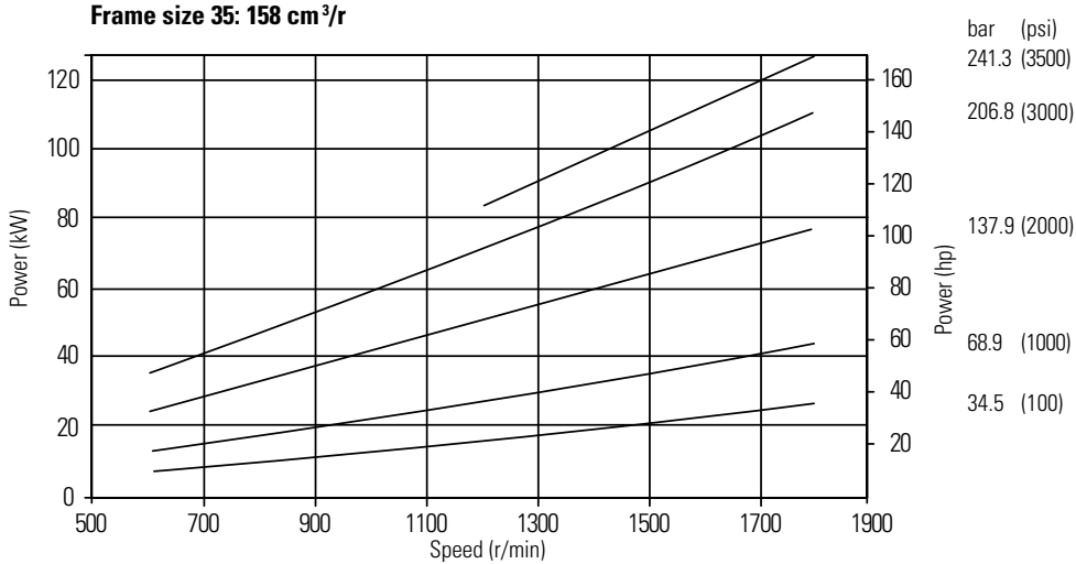
Frame size 35: 158 cm 3 /r
