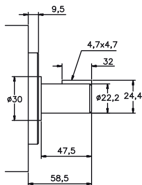
Nº1 Shaft
