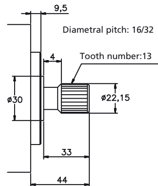
Nº2 Shaft
