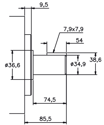
N°86 Shaft
