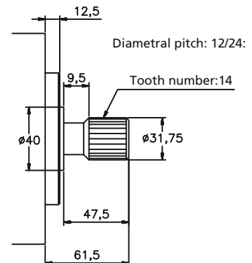
N°2 Shaft
