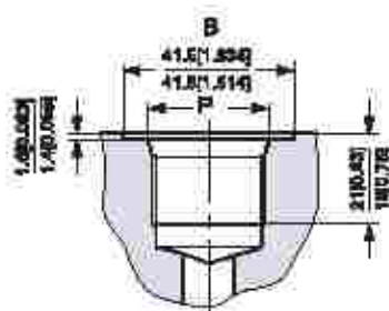
B: UNF Main port P: 1 1/8 – 12 UN
