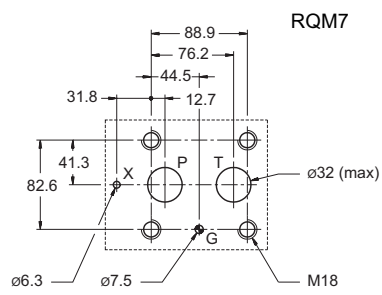
ISO 6264-10-17-*97 (CETOP 4.4.2-2-R10-350)
