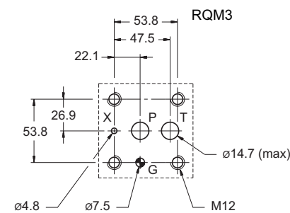
ISO 6264-06-09-*97 (CETOP 4.4.2-2-R06-350)
